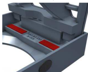
Csuklópánt és HYDROpren csillapító betét
