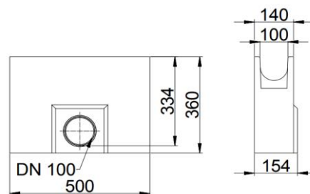
Iszapfogó akna
