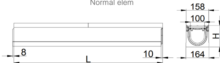
Normál elem
