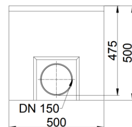
Iszapfogó akna
