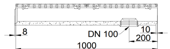
Kifolyós elem
