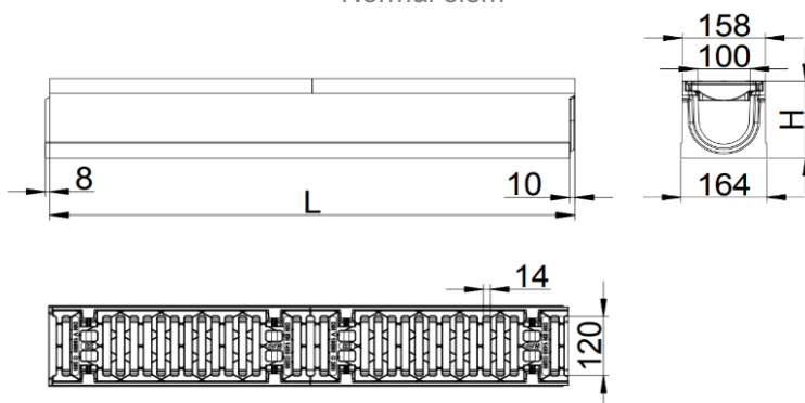
Normál elem
