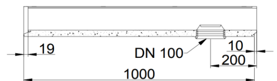
Kifolyós elem
