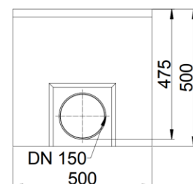
Iszapfogó akna
