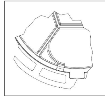
Rugókaros zárszerkezet - részlet
